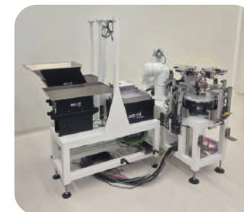
Charlie Robot de remplissage pour le produit 4DryField®
